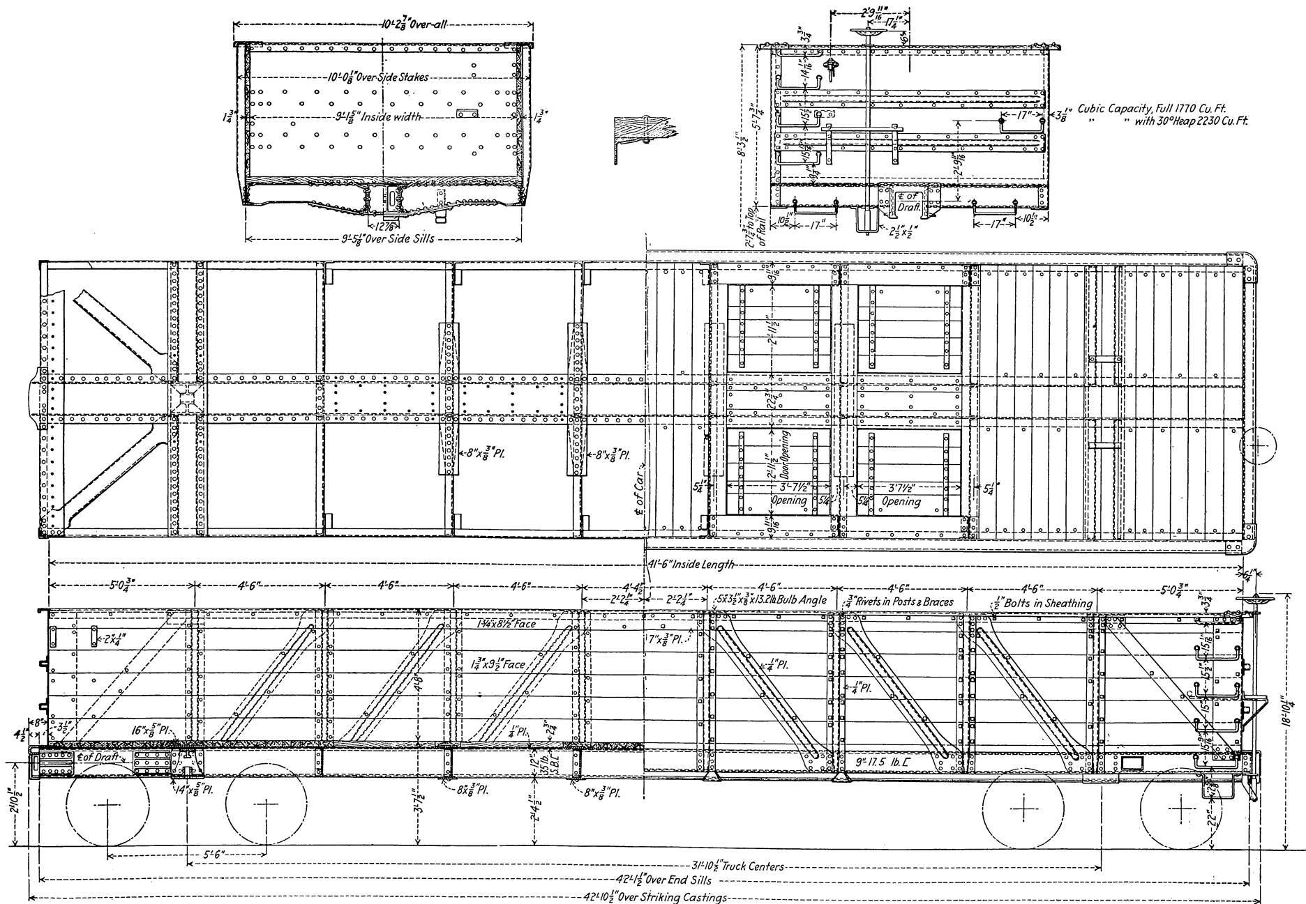
Fig. 2868—U. S. R. A. Standard, Composite 50-Ton Gondola Cor. (See Figs. 2848 and 2869.)
